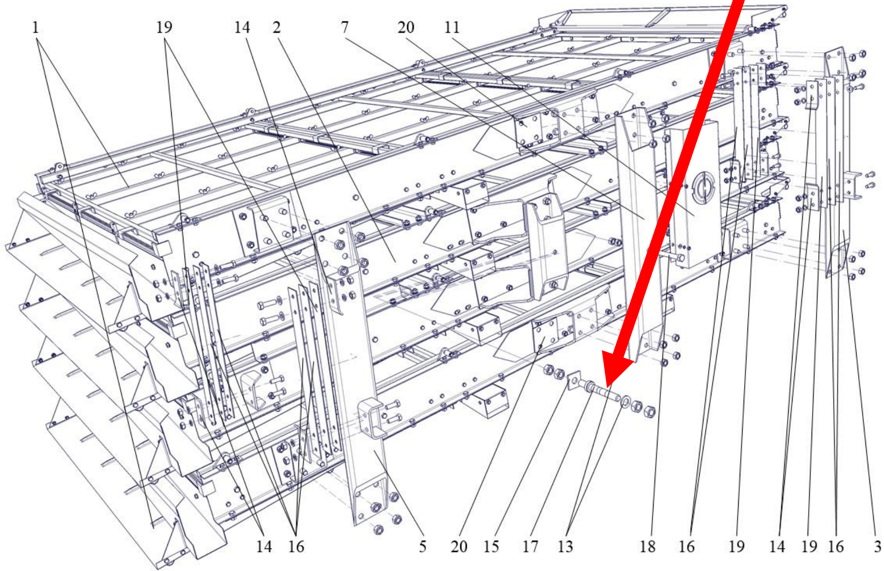
Рис. 12 СВУ60.07.000А
